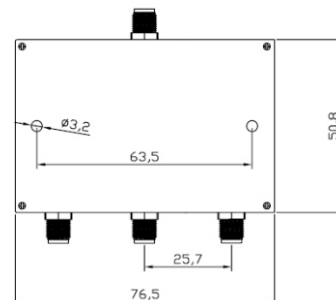
外形图
