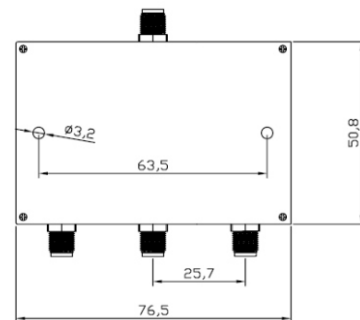
外形图
