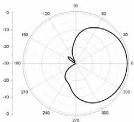
H-Plane
