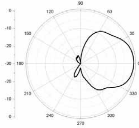
E-Plane
