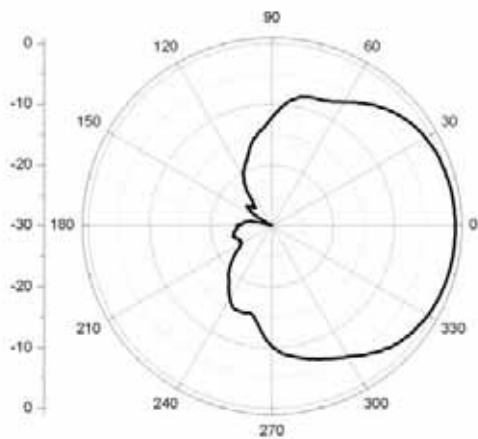
H-Plane
