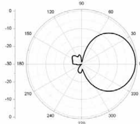
E-Plane
